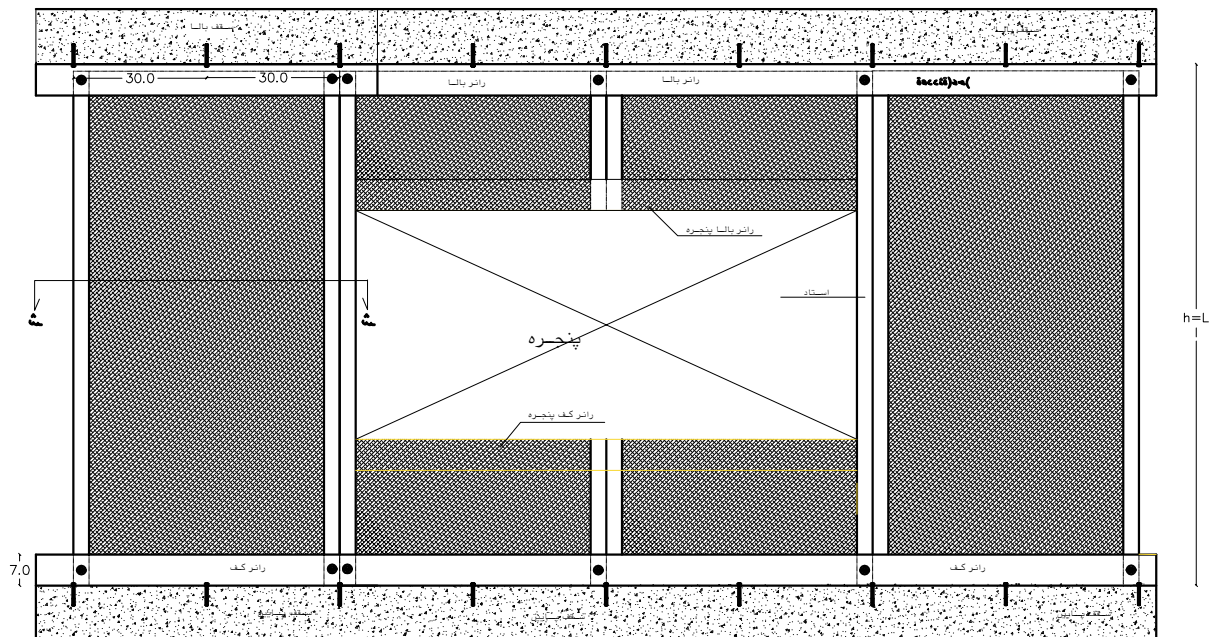
جزییات دیوار شیلر بازشو
